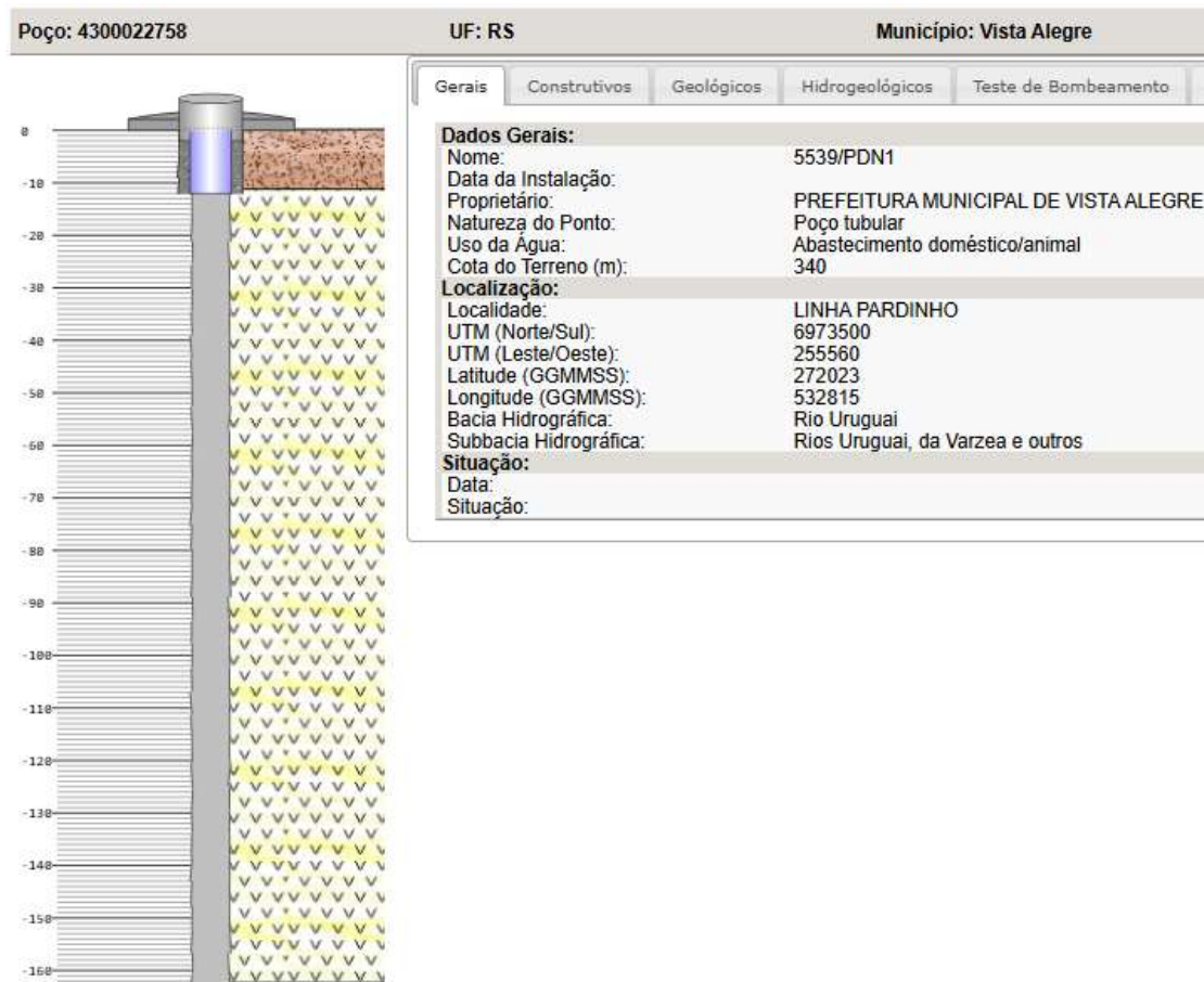
Figura 12: Perfil Geológico do Poço 2. Fonte: SIAGAS (2025).
