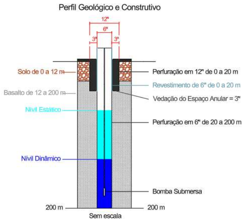
Figura 13: Perfil Geológico e Construtivo do Poço. Fonte: Autor (2025).
